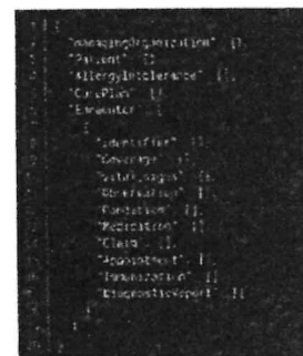
โครงสร้างมาตรฐานที่ปรับปรุงมาจาก HL7 FHIR โดยการส่งข้อมูลจะถูกจัดเก็บในรูปแบบของ JSON
