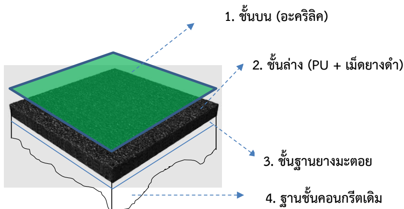
รูปที่ ๑ แสดงตัวอย่างองค์ประกอบของแผ่นพื้นสนามกีฬา
