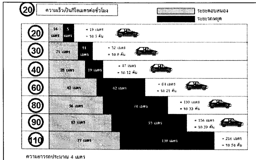
รูปที่ ๒ ระยะหยุดที่ความเร็วแตกต่างกัน
