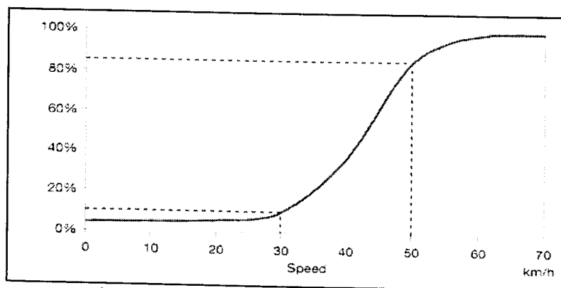
รูปที่ ๑ โอกาสเสียชีวิตเนื่องจากแรงกระแทกในการชนของรถ
